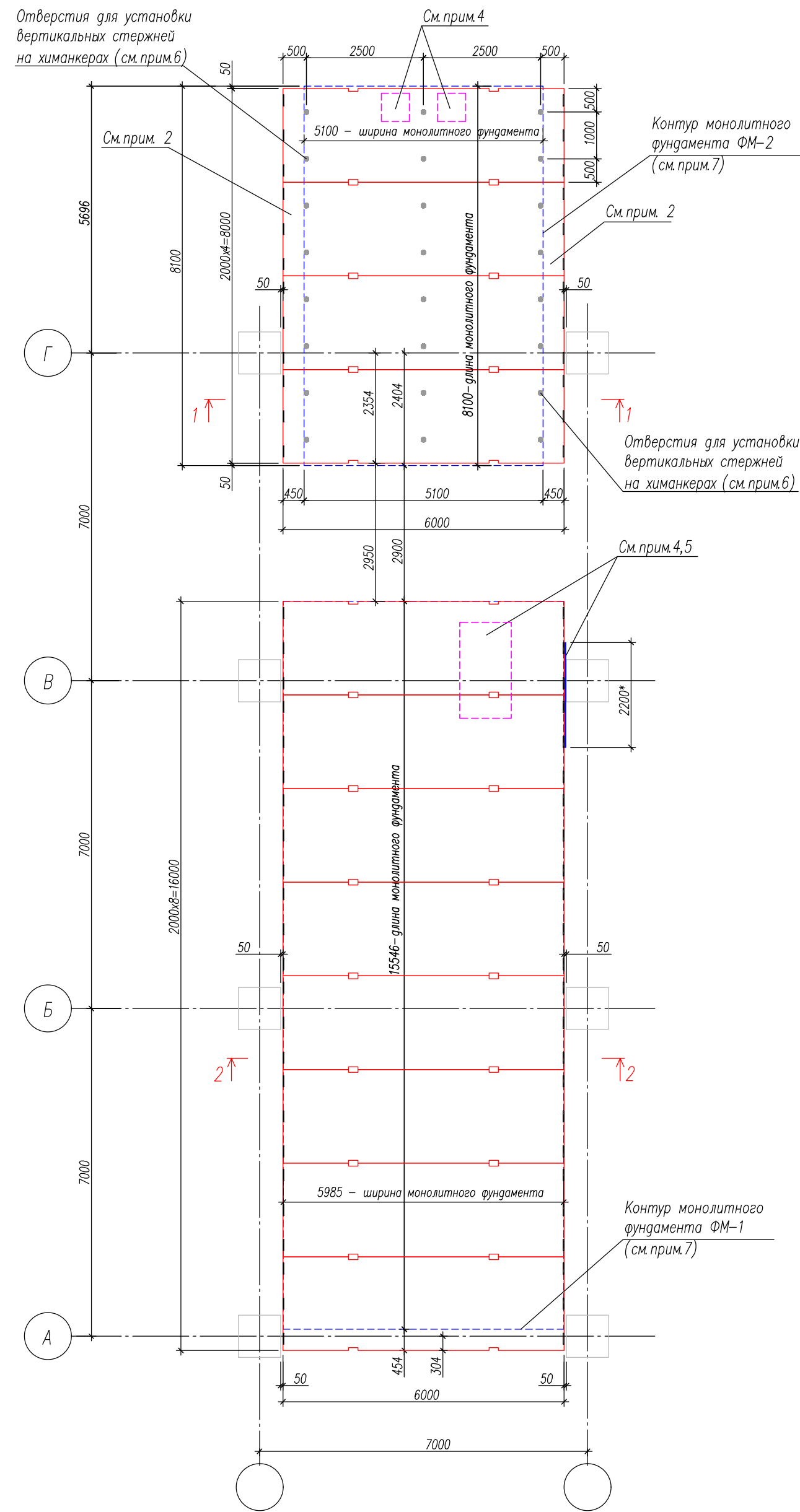
Схема раскладки 2-го ряда ПАГ 18 для устройства сборных фундаментов под энергомодули и ДГУ
