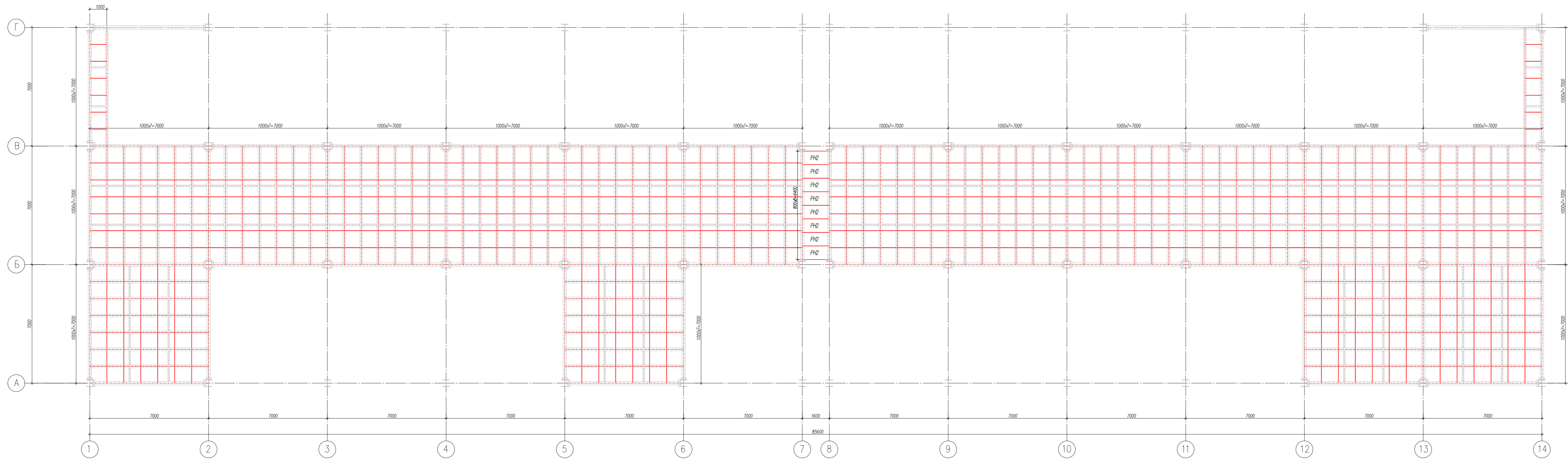
Схема раскладки щитов сварного решетчатого настила на отм. 4,900.
