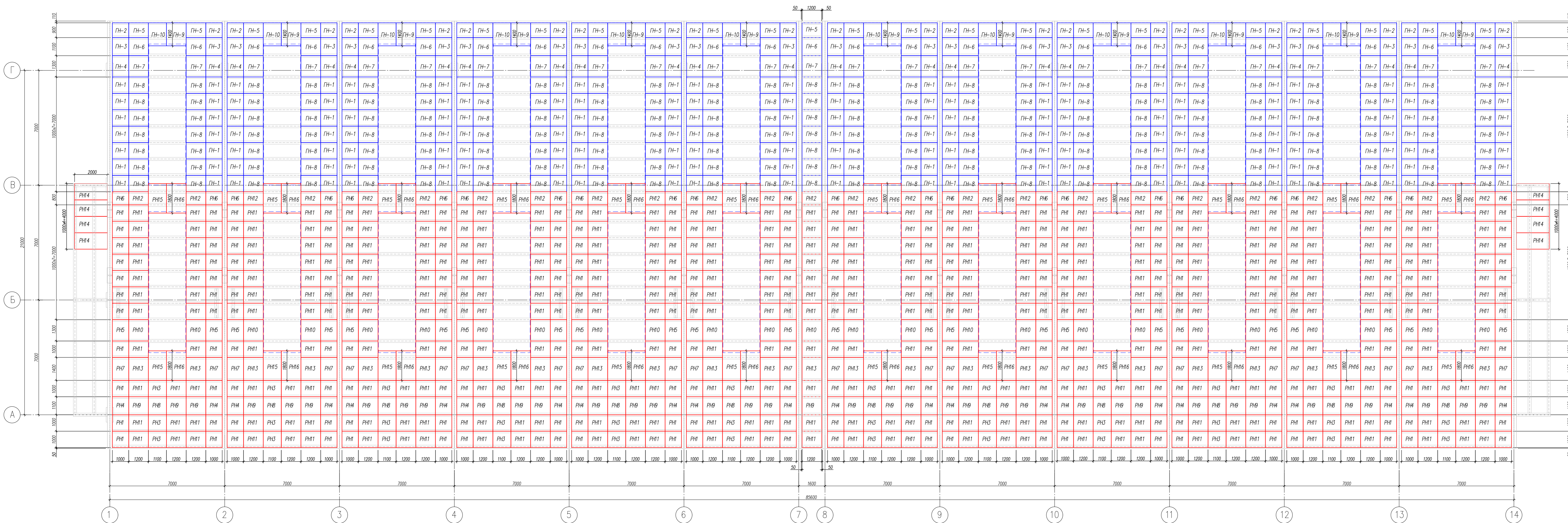
Схема раскладки щитов сварного решетчатого настила на отм. 7,407.
