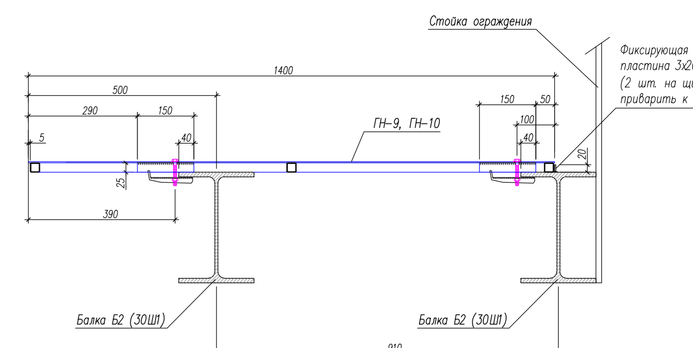
Узел крепления щитов глухого настила РН-9, РН-10
