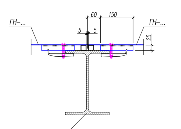
Узел крепления щитов глухого настила
